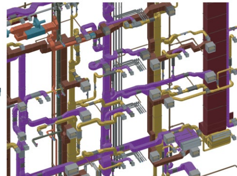
Abb. 3: Ausführungsplanung KG 430
