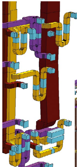
Abb. 2: Entwurfsplanung
